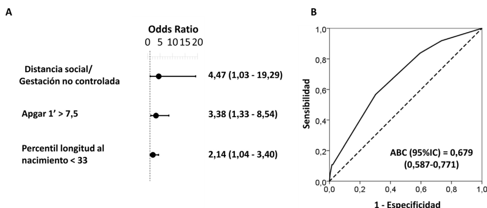
Figura 2 [vs2] Regresión binaria logística de los factores de riesgo asociados a toxicología positiva de de los neonatos mayores a 34 SG ingresados en UCIN y UCMN. Forest plot (A) y curva ROC (B) del modelo multivariante obtenido. En la tabla se indican las odds ratio (OR) crudas y ajustadas con sus intervalos de confianza entre paréntesis. Los valores de punto corte óptimos fueron determinados por el índice máximo de Youden (J), definido como (sensibilidad + especificidad - 1). La comparación de las frecuencias esperadas y observadas se realizó por la prueba de bondad de ajuste Hosmer-Lemeshow ( p = 0,983 ) y por su curva ROC y su área bajo la curva (ABC), indicando un buen ajuste para el modelo.
